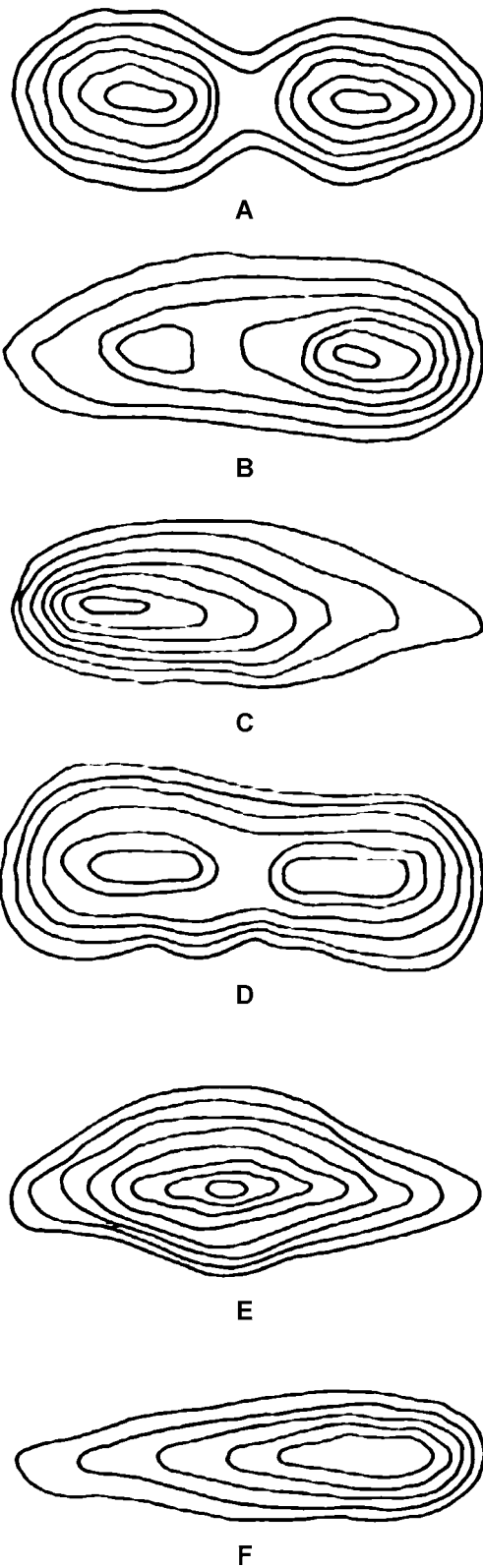
Figure B-2 Exemples de caractéristiques des courbes D Cad 3, 2007, Ottawa ON, Ministère de la Défense nationale
